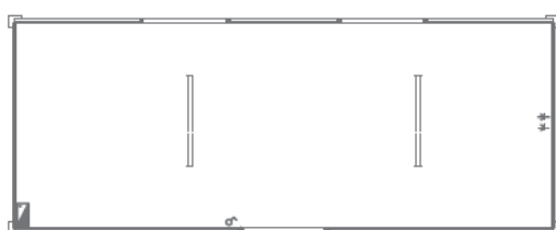
▲ 1142 kancelarijski, 6,0 x 2,4 m, jedna vrata, 2 prozora, termoizolovan, razvod struje nazidno PVC kanalicama, osigurači, dve fluo baterije 2 x 36W IP 54, dve monofazne utičnice, pod laminat
