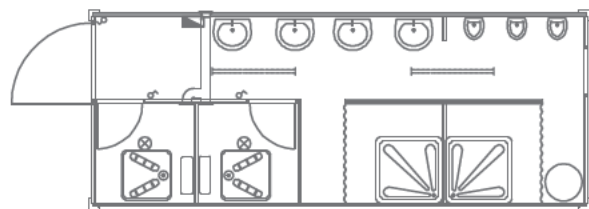
▲ 1145 sanitarni kontejner dimenzija 6,0 x 2,4 m 4 umivaonika, 3 pisoara, 2 WC kabine, 2 tuš kabine, termoizolovan, boiler, pod keramika, razvod struje nazidno PVC kanalicama, osigurači, dve fluo baterije 2 x 36W IP 54, dve monofazne utičnice, prozor,
