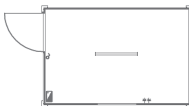
▲ 1132 kancelarijski kontejner 3,6 x 2,4 m 1 vrata, 1 prozor, termoizolovan, razvod struje razvod struje nazidno PVC kanalicama, osigurači, fluo baterija 2 x 36W IP 54, dve monofazne utičnice, pod laminat
