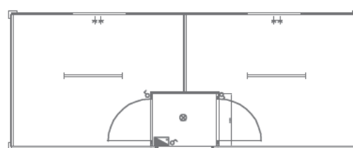
▲ 1141 kancelarijski, 6,0 x 2,4 m, podeljen na dve prostorije i pretprostor, 3 vrata, 2 prozora, termoizolovan, pod laminat, razvod struje nazidno PVC kanalicama, osigurači, dve fluo baterije 2 x 36W IP 54 i plafonjera, 4 monofazne utičnice, pod laminat
