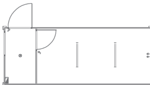
▲ 1104 kancelarijski kontejner 6,0 x 2,4 m sa pretprostorom, 2 vrata, 3 prozora, termoizolovan, razvod struje nazidno PVC kanalicama, osigurači, dve fluo baterije 2 x 36W IP 54, dve monofazne utičnice, pod laminat
