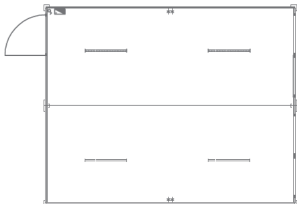
▲ 1162 kancelarijski sklop 6,0 x 4,8 m termoizolovan, vrata, 4 prozora, razvod struje nazidno PVC kanalicama, osigurači, 4 fluo baterije 2 x 36W IP 54, 4 monofazne utičnice, osigurači, pod laminat
