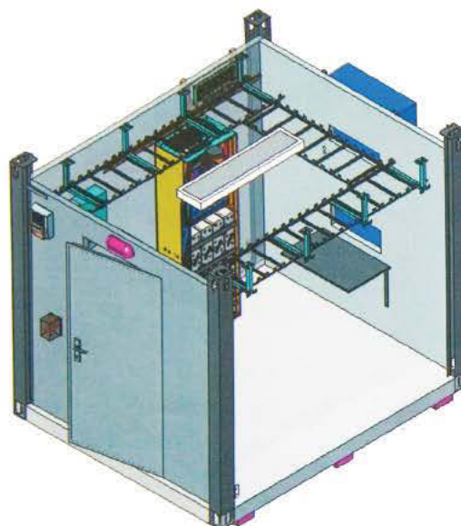
▼ 3D prikaz unutrašnje opreme kontejnera
