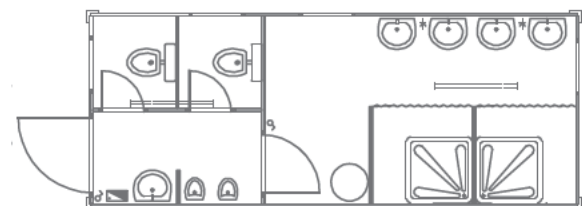
▲ 1108 sanitarni kontejner 6,0 x 2,4 m 2 WC kabine, 5 umivaonika, 2 pisoara, bojler, 2 tuš kabine, 4 prozora, termoizolovan, razvod struje nazidno PVC kanalicama, osigurači, dve fluo baterije 2 x 36W IP 54, dve monofazne utičnice,
