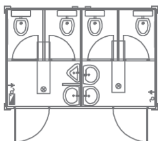
▲ 1174 sanitarni 3,5 x 2,4 m, termoizolovan, u dva prostora (M / Ž), 6 vrata, 3 umivaonika, pisoar, 4 WC kabine, razvod struje nazidno PVC kanalicama, osigurači, 2 fluo baterije 2 x 36W IP 54, 2 monofazne utičnice, osigurači, pod keramika
