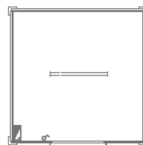
◀ 1146 skladišni kontejner 2,4 x 2,4 m, termoizolovan, vrata, razvod struje nazidno PVC kanalicama, osigurači, dve fluo baterije 2 x 36W IP 54, dve monofazne utičnice, pod vodootporna iverica
