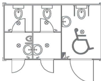
▲ 1175 sanitarni kontejner 4,2 x 2,4 m termoizolovan, u tri prostora (M / Ž / I), 5 vrata, 3 umivaonika, pisoar, 3 WC kabine, razvod struje nazidno PVC kanalicama, osigurači, 3 fluo baterije 2 x 36W IP 54, 3 monofazne utičnice, osigurači, pod keramika
