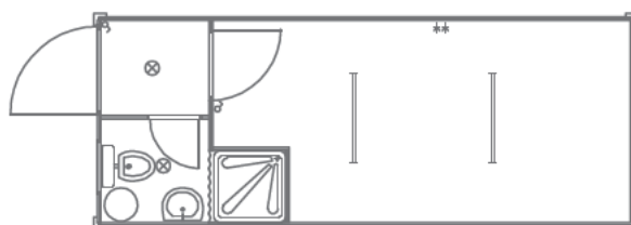
▲ 1106 kancelarijski kontejner 6,0 x 2,4 m sa pretprostorom i opremljenom sanitarijom sa tušem, 2 vrata, 3 prozora, termoizolovan, razvod struje nazidno PVC kanalicama, osigurači, dve fluo baterije 2 x 36W IP 54, dve monofazne utičnice, pod laminat
