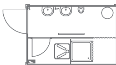
▲ 1143 sanitarni kontejner 3,0 x 2,4 m termoizolovan, pod keramika, 2 vrata, 2 umivaonika, tuš kabina, pisoar, WC kabina, boiler, razvod struje nazidno PVC kanalicama, osigurači, fluo baterija 2 x 36W IP 54, dve monofazne utičnice, prozor
