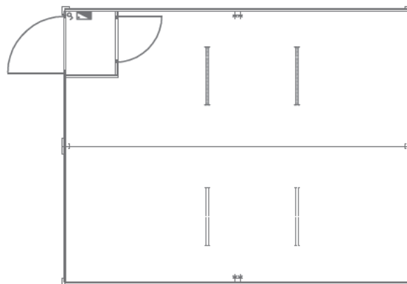
▲ 1163 kancelarijski sklop 6,0 x 4,8 m sa pretprostorom, termoizolovan, 2 vrata, 4 prozora, razvod struje nazidno PVC kanalicama, osigurači, 4 fluo baterije 2 x 36W IP 54, 4 monofazne utičnice, osigurači, pod laminat
