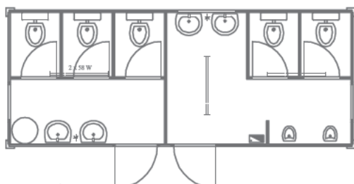
▲ 1107 sanitarni kontejner 6,0 x 2,4 m Ženski i muški deo: ukupno 5 WC kabina, 4 umivaonika, 2 pisoara, 2 prozora, jedan bojler, pod keramika, termoizolovan, razvod struje nazidno PVC kanalicama, osigurači, dve fluo baterije 2 x 36W IP 54, dve monofazne utičnice,
