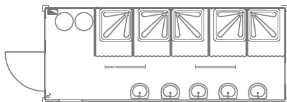
▲ 1109 sanitarni kontejner 6,0 x 2,4 m 5 umivaonika, 5 tuš kabina, dva bojlera, pod keramika, 3 prozora, termoizolovan, razvod struje nazidno PVC kanalicama, osigurači, dve fluo baterije 2 x 36W IP 54, dve monofazne utičnice
