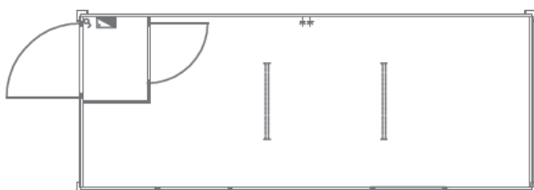
▲ 1103 kancelarijski kontejner 6,0 x 2,4 m sa pretprostorom, 2 vrata, 2 prozora, termoizolovan, razvod struje nazidno PVC kanalicama, osigurači, dve fluo baterije 2 x 36W IP 54, dve monofazne utičnice, pod laminat
