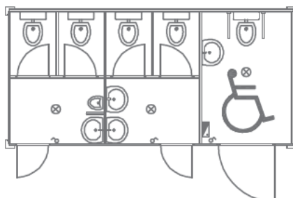
▲ 1176 sanitarni 6,0 x 2,4 m 6,0 x 2,4 m, termoizolovan, u tri prostora (M / Ž / I), 7 vrata, 4 umivaonika, pisoar, 5 WC kabina, razvod struje nazidno PVC kanalicama, osigurači, 3 fluo baterije 2 x 36W IP 54, 4 monofazne utičnice, osigurači, pod keramika
