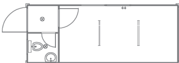
▲ 1105 kancelarijski kontejner 6,0 x 2,4 m sa pretprostorom i opremljenom sanitarijom, 2 vrata, 3 prozora, termoizolovan, razvod struje nazidno PVC kanalicama, osigurači, dve fluo baterije 2 x 36W IP 54, dve monofazne utičnice, pod laminat
