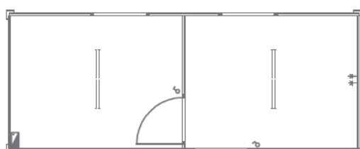
▲ 1137 kancelarijski, 6,0 x 2,4 m podeljen na dve prostorije, 2 vrata, 2 prozora, termoizolovan, pod laminat, razvod struje nazidno PVC kanalicama, osigurači, dve fluo baterije 2 x 36W IP 54, 4 monofazne utičnice, pod laminat
