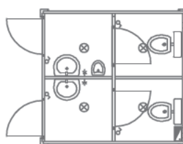
▲ 1173 sanitarni, 2,6 x 2,4 m termoizolovan, u dva prostora (M / Ž), 4 vrata, 2 umivaonika, pisoar, 2 WC kabine, razvod struje nazidno PVC kanalicama, osigurači, 3 fluo baterije 2 x 36W IP 54, 2 monofazne utičnice, osigurači, pod keramika
